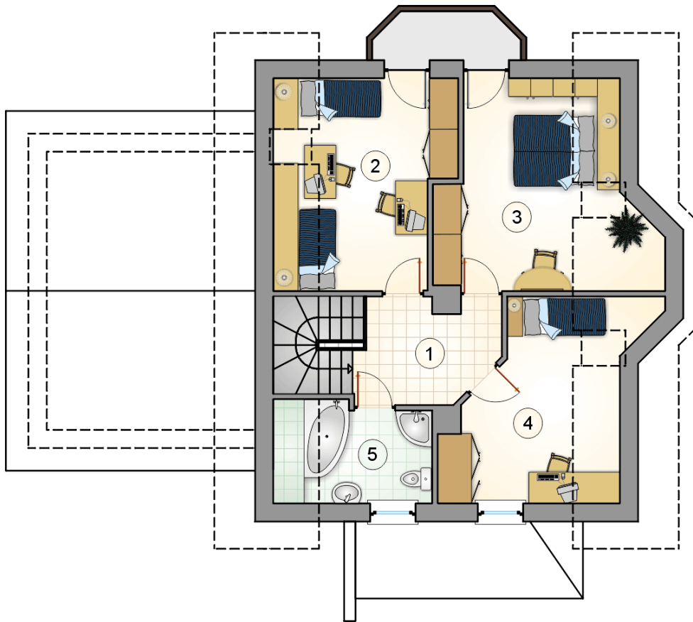
RZUT PODDASZA
