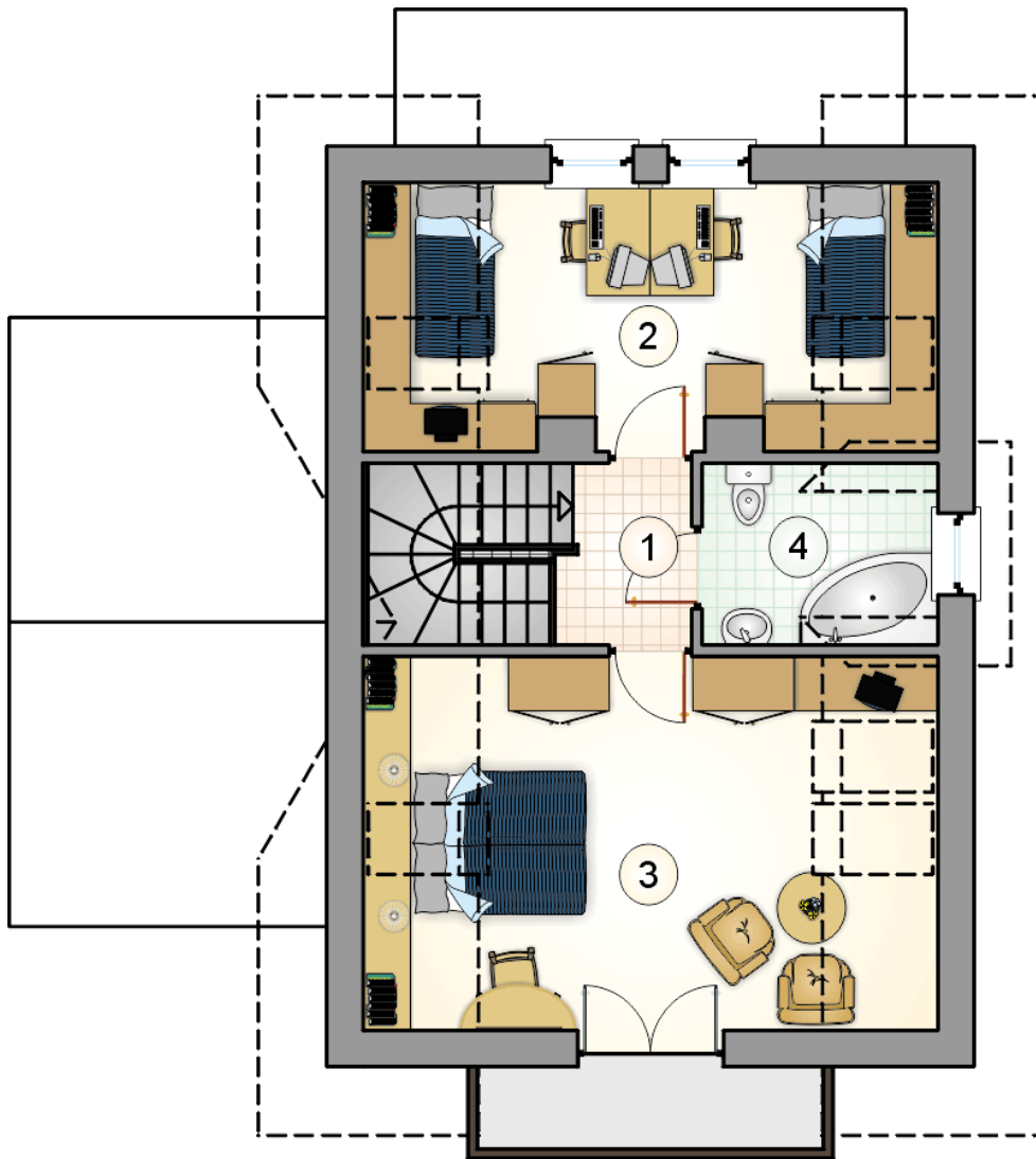
RZUT PODDASZA
