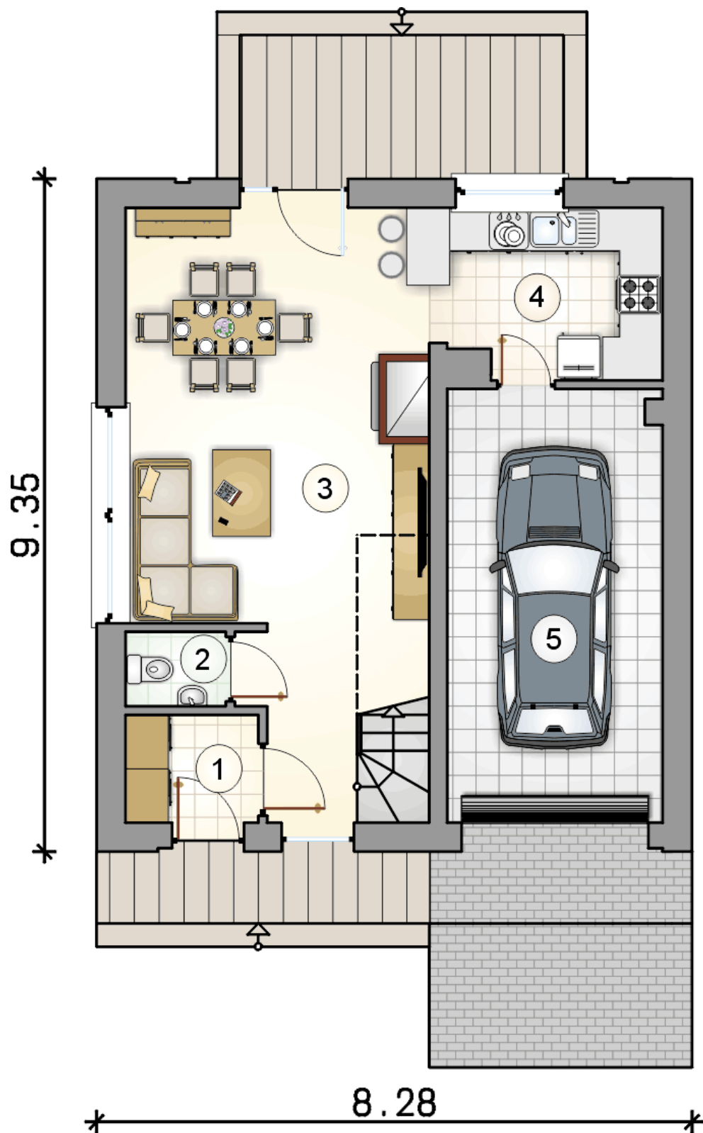
RZUT PARTERU
