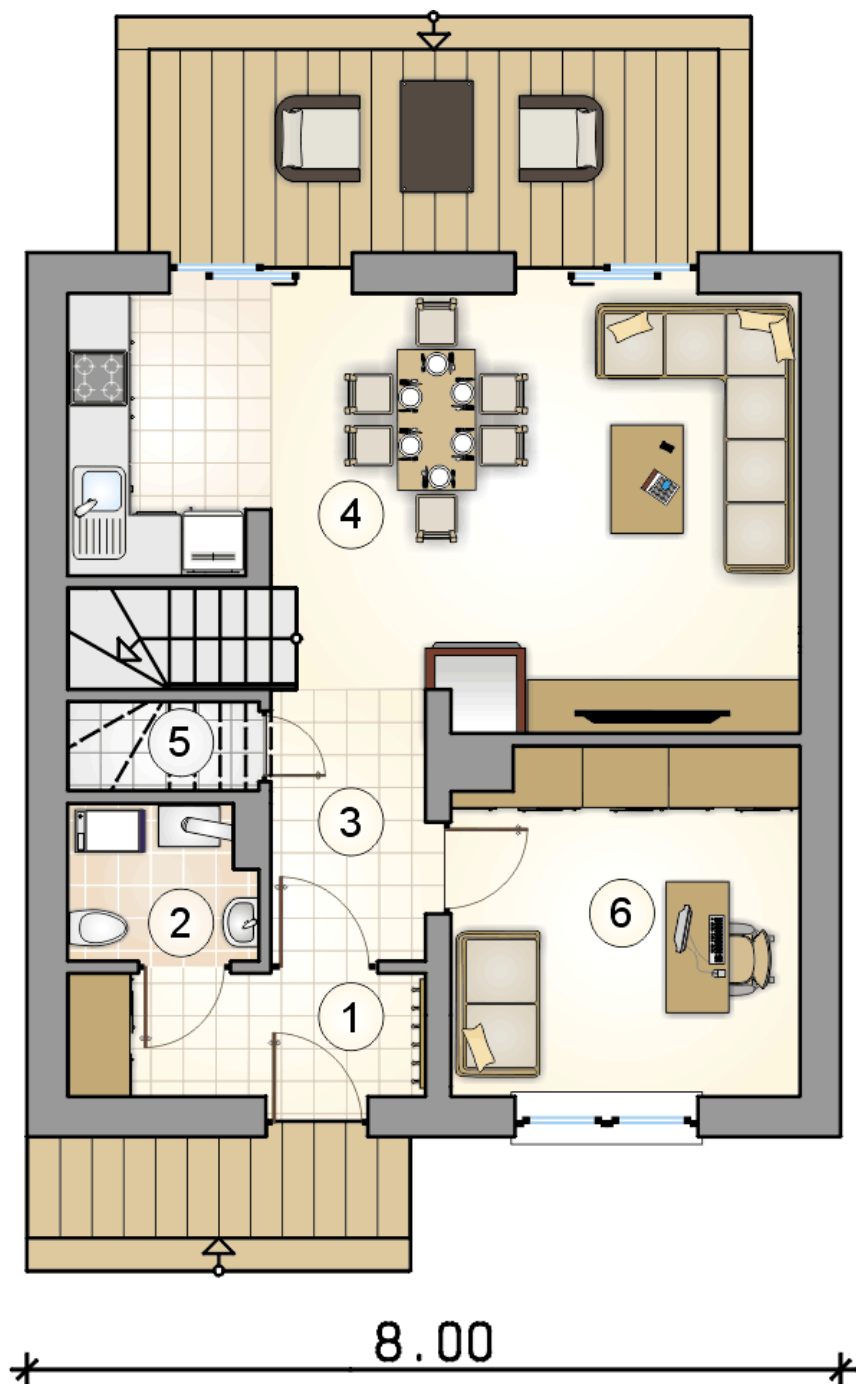
RZUT PARTERU
