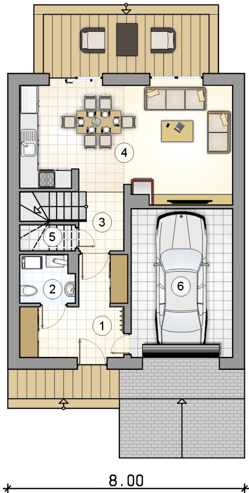
RZUT PARTERU
