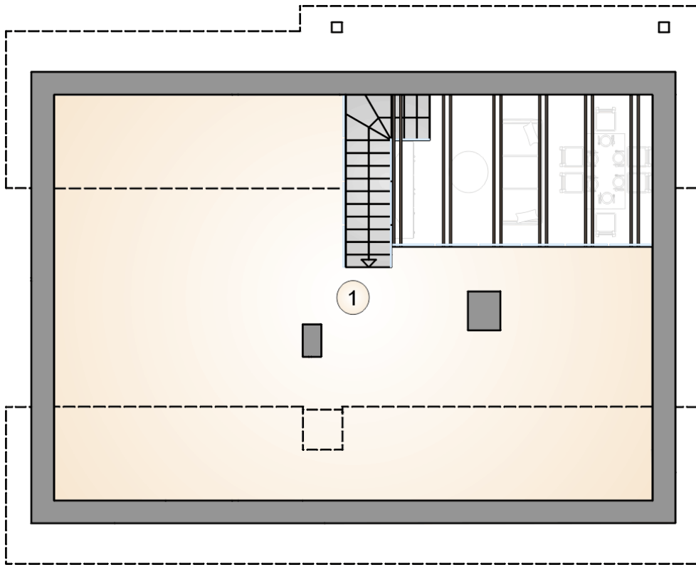
RZUT PODDASZA
