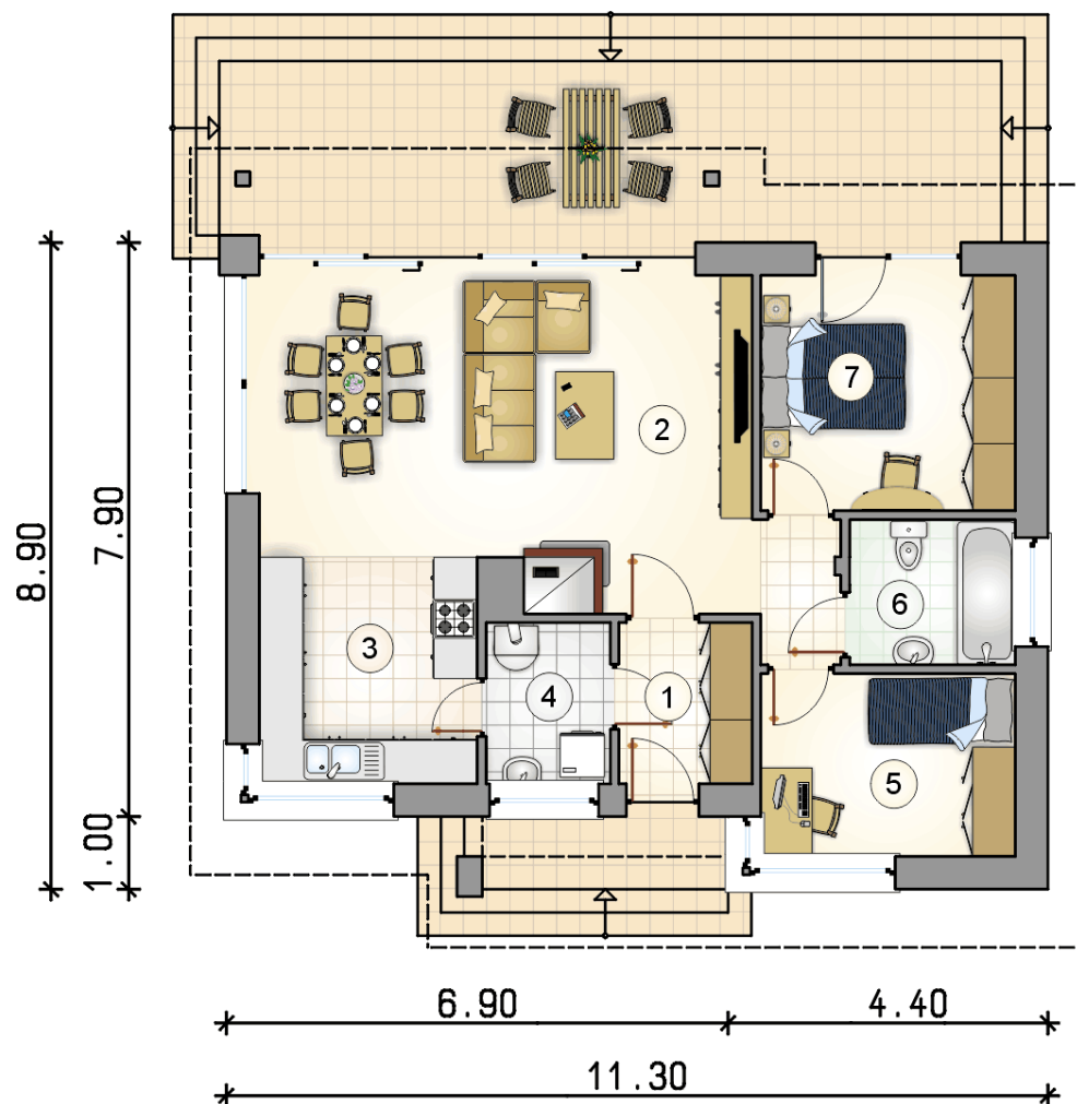
RZUT PARTERU
