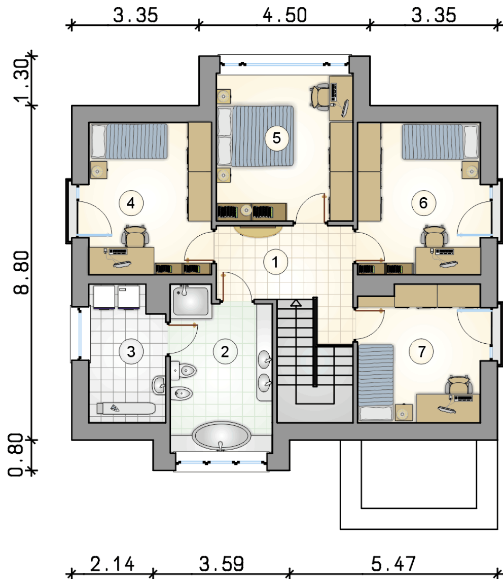
RZUT PIĘTRA
