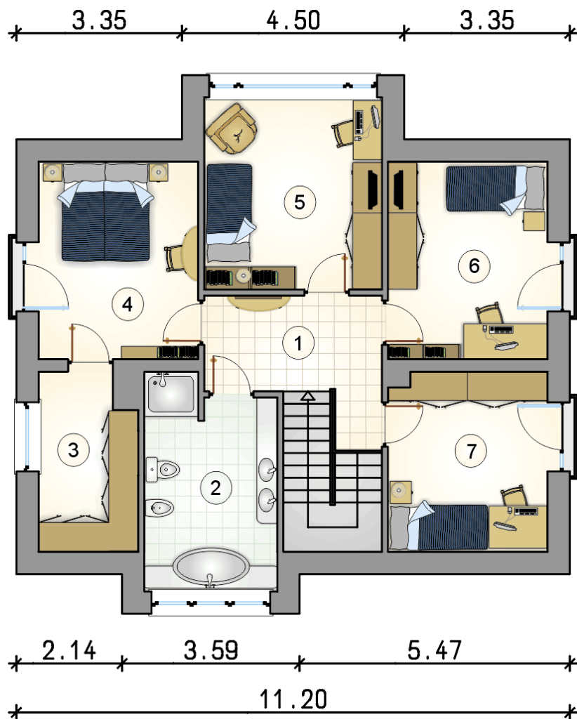
RZUT PIĘTRA
