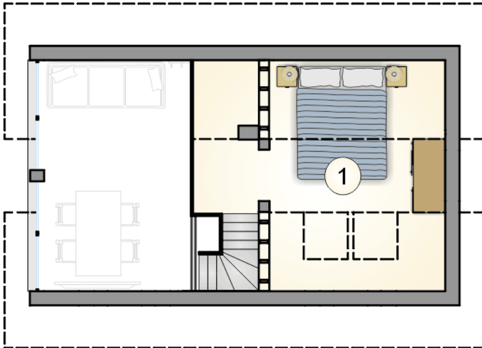
RZUT PODDASZA
