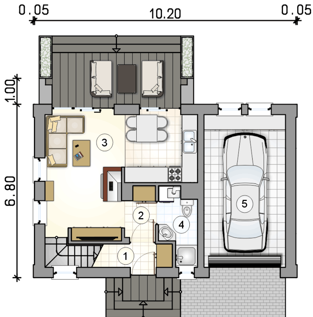
RZUT PARTERU
