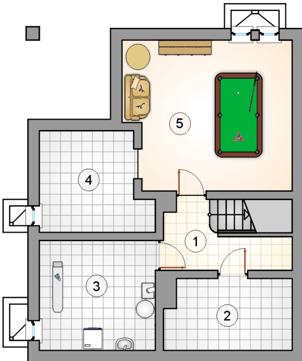
RZUT PIWNICY
