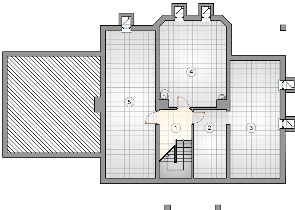
RZUT PIWNICY
