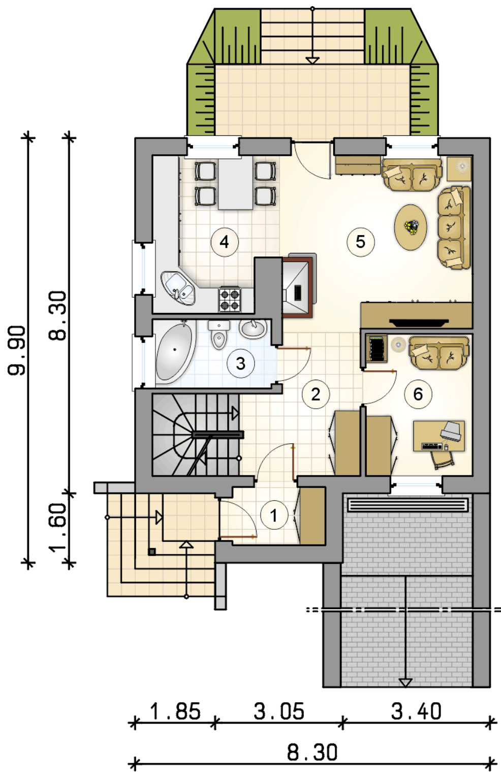
RZUT PARTERU
