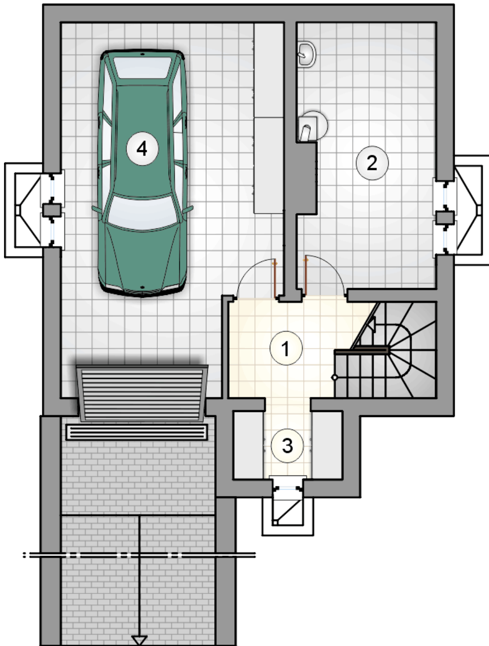
RZUT PIWNICY
