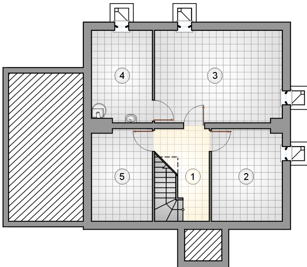
RZUT PIWNIC
