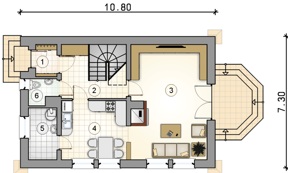
RZUT PARTERU
