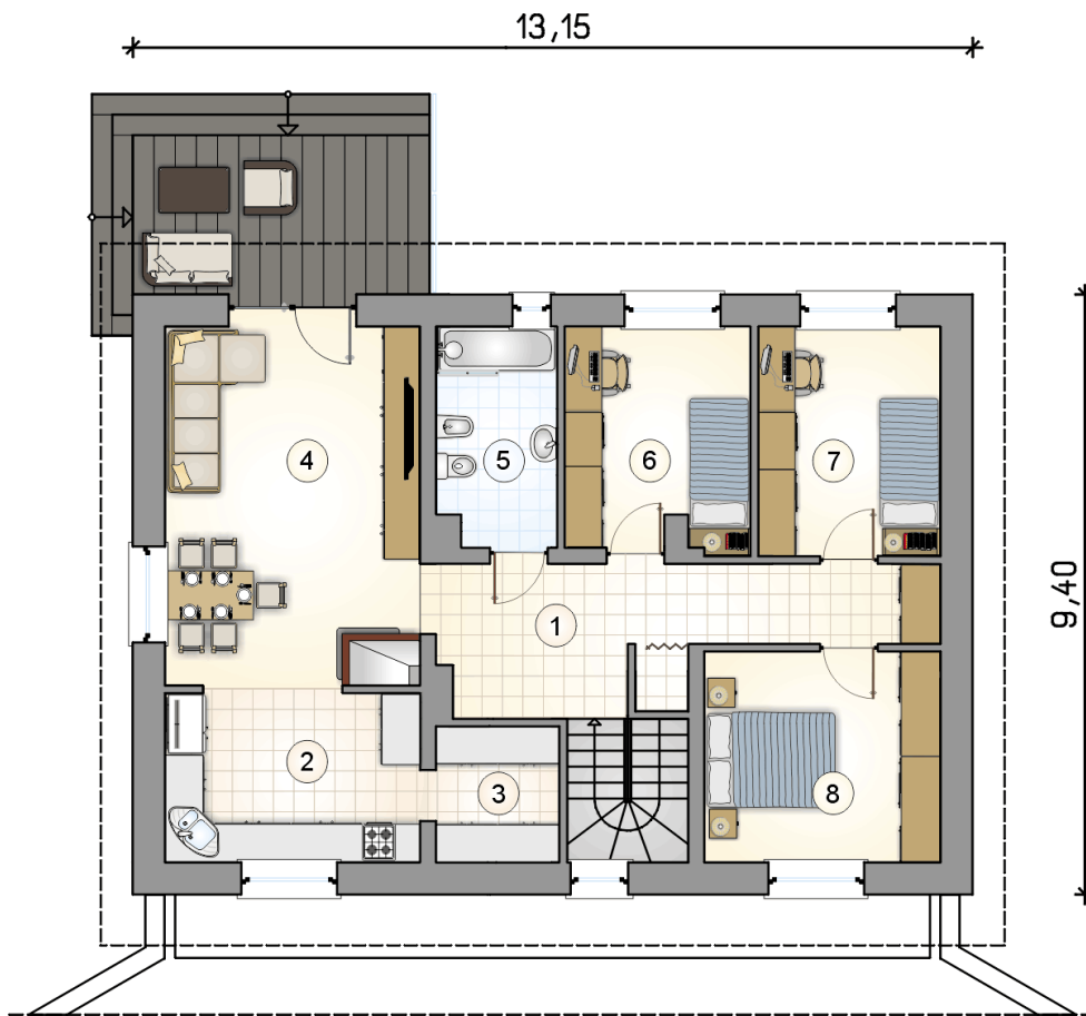
RZUT PARTERU
