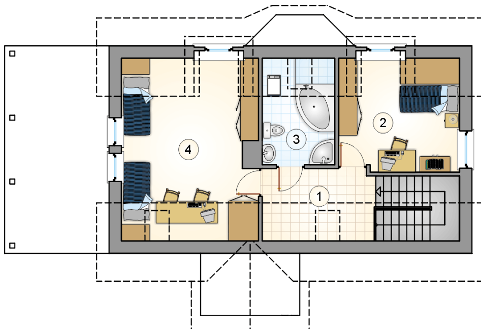
RZUT PODDASZA
