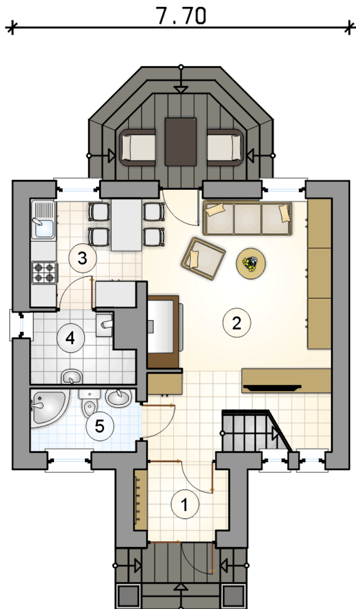
RZUT PARTERU
