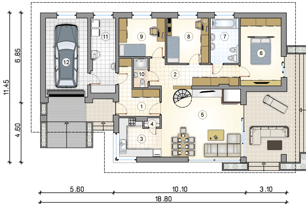
RZUT PARTERU PROJEKTU KOS VII
