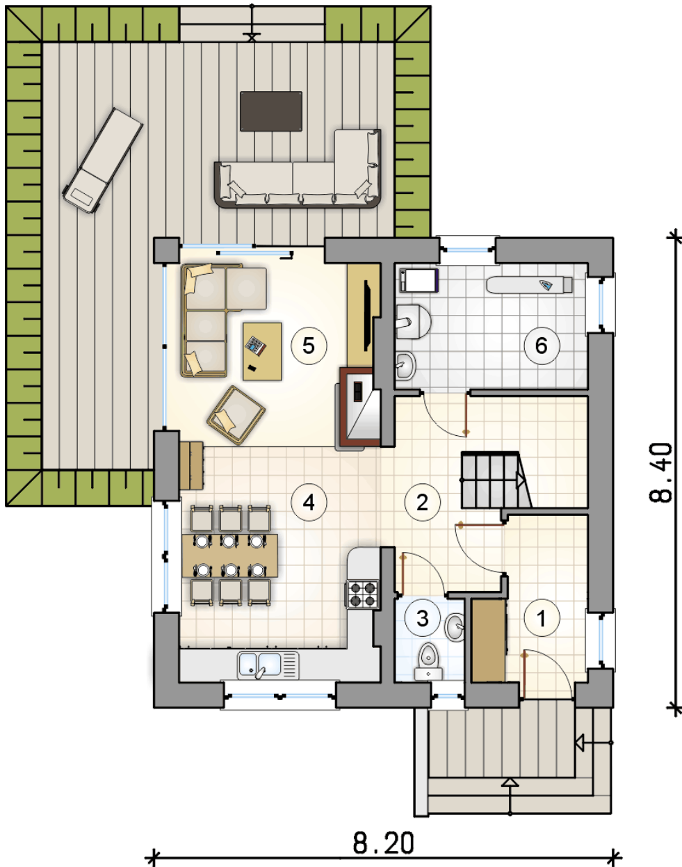
RZUT PARTERU
