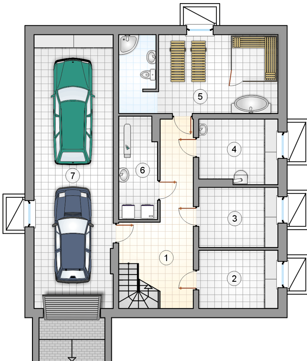
RZUT PIWNICY
