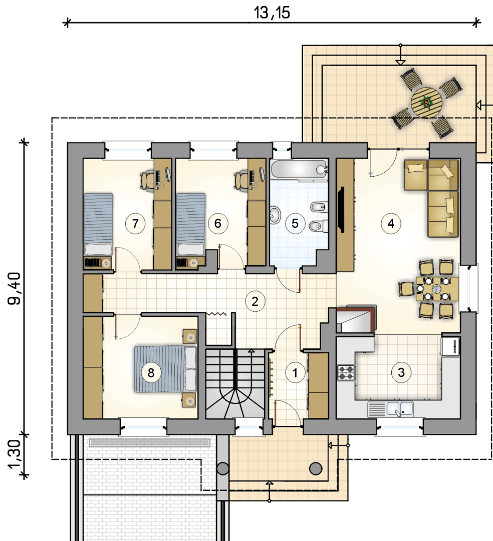
RZUT PARTERU
