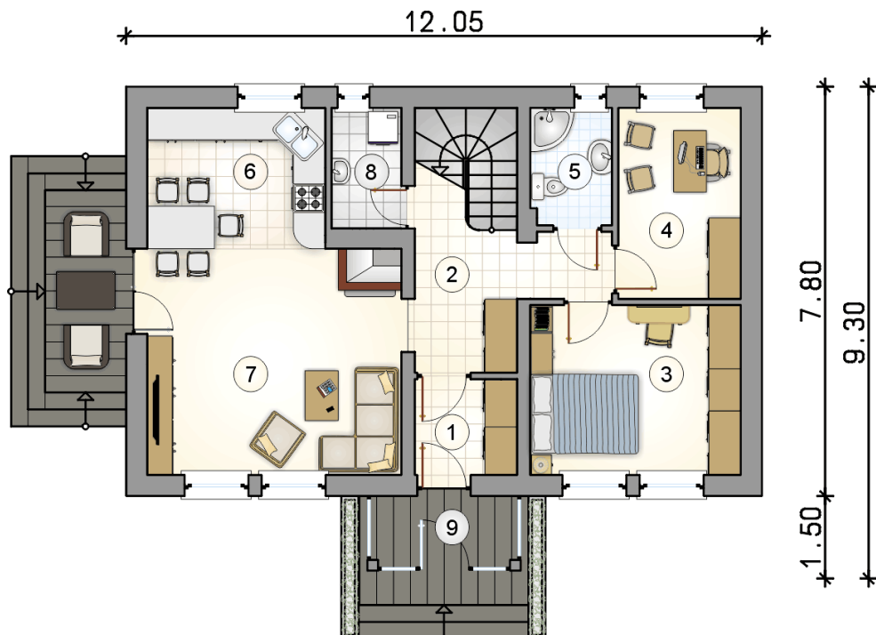
RZUT PARTERU
