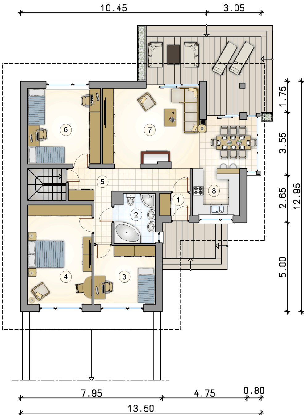
RZUT PARTERU
