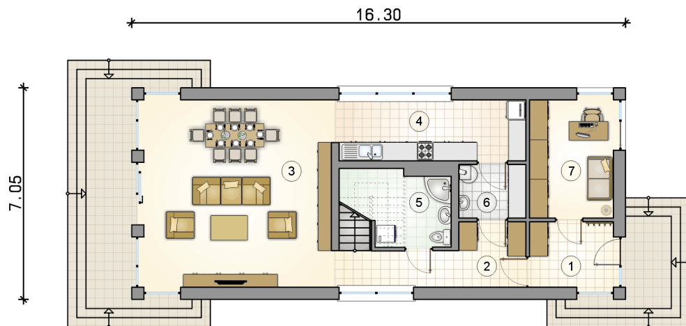
RZUT PARTERU PROJEKTU GARDA III [m 2 ]
