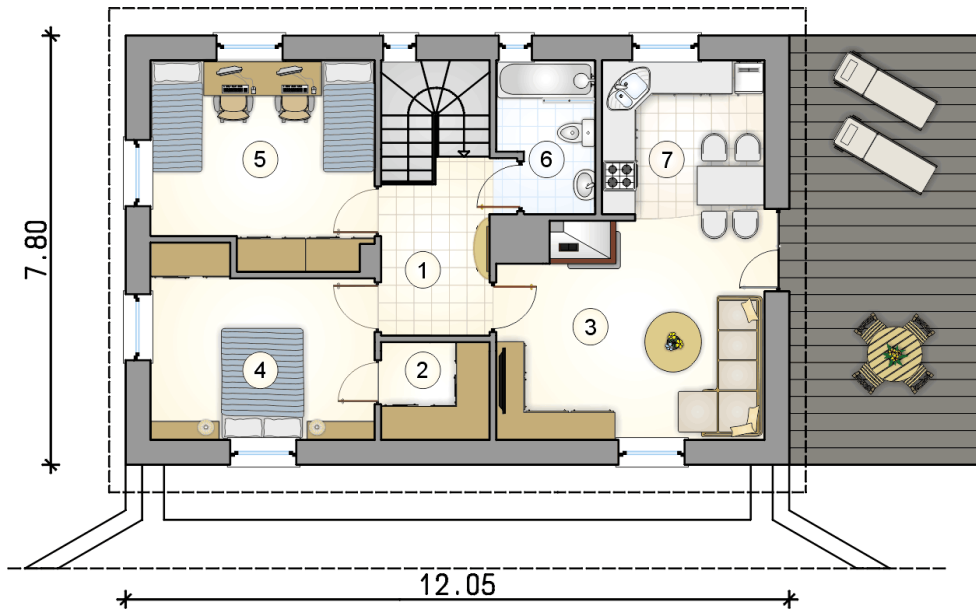
RZUT PARTERU
