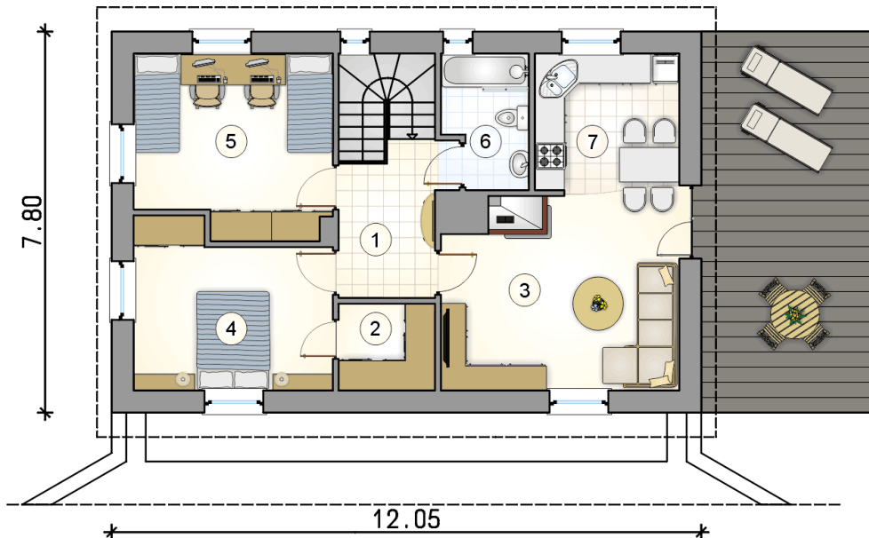
RZUT PARTERU
