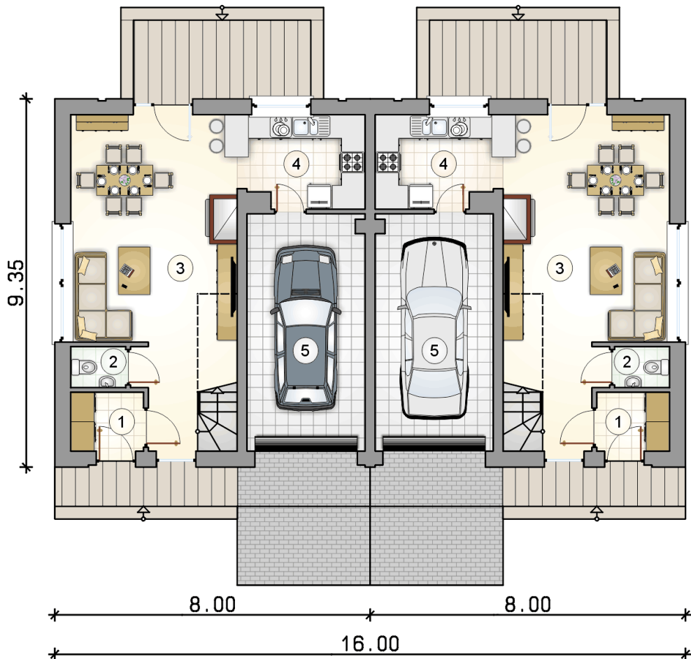
RZUT PARTERU
