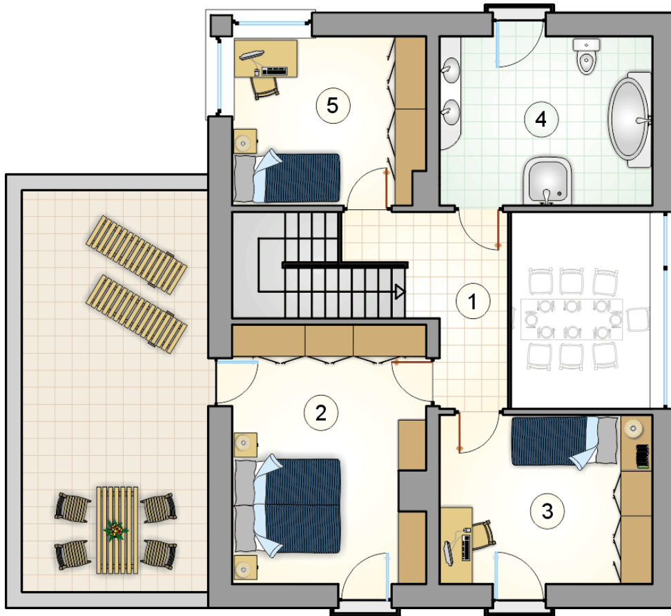
RZUT PIĘTRA
