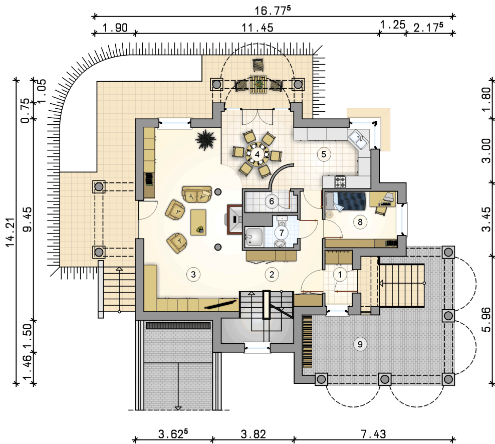
RZUT PARTERU
