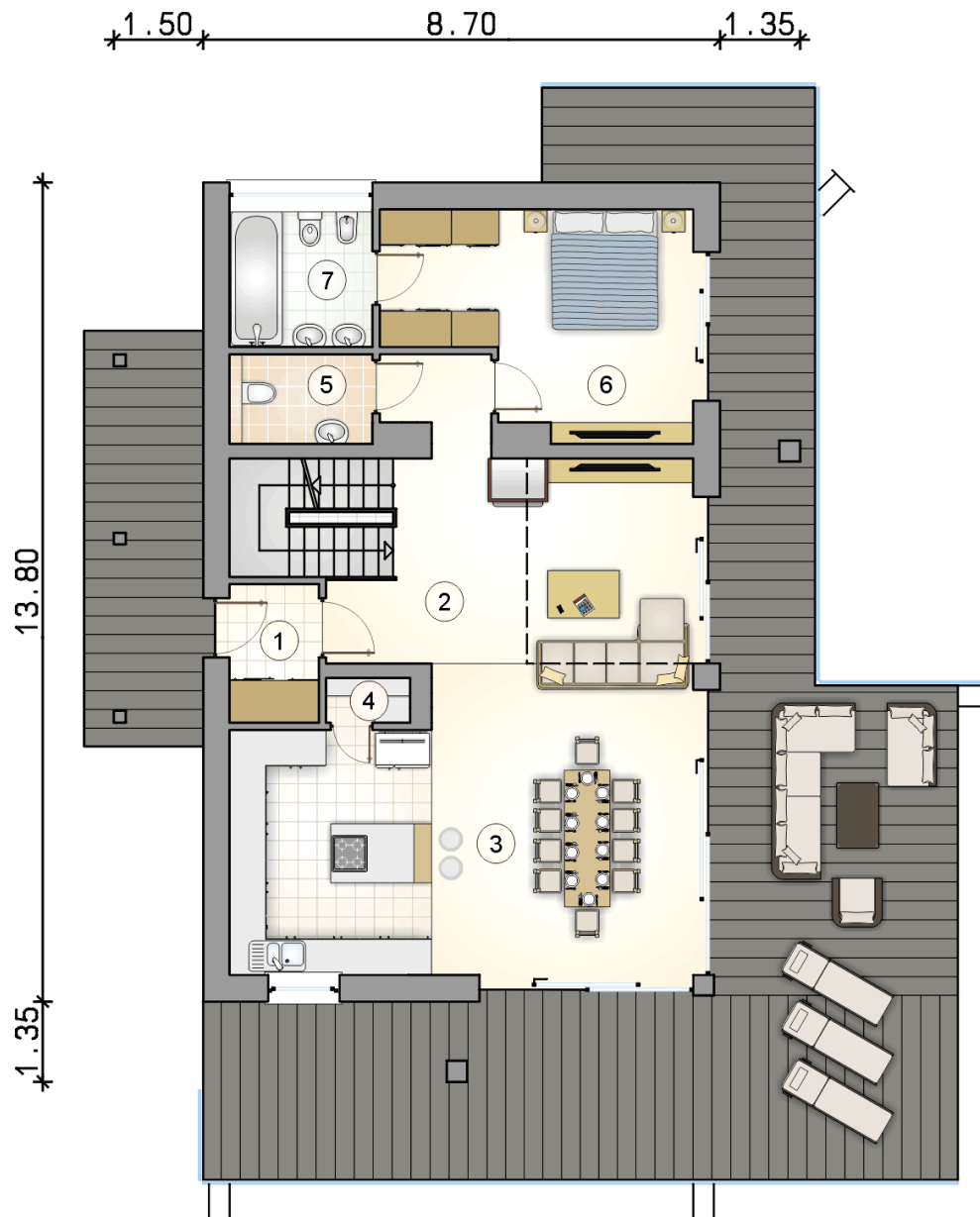
RZUT PARTERU
