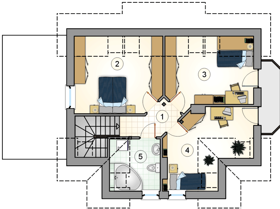
RZUT PODDASZA
