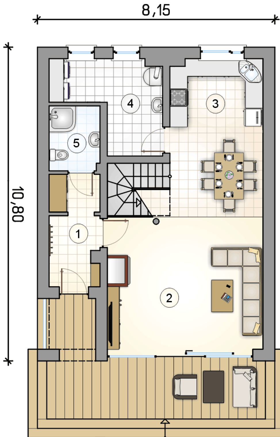
RZUT PARTERU
