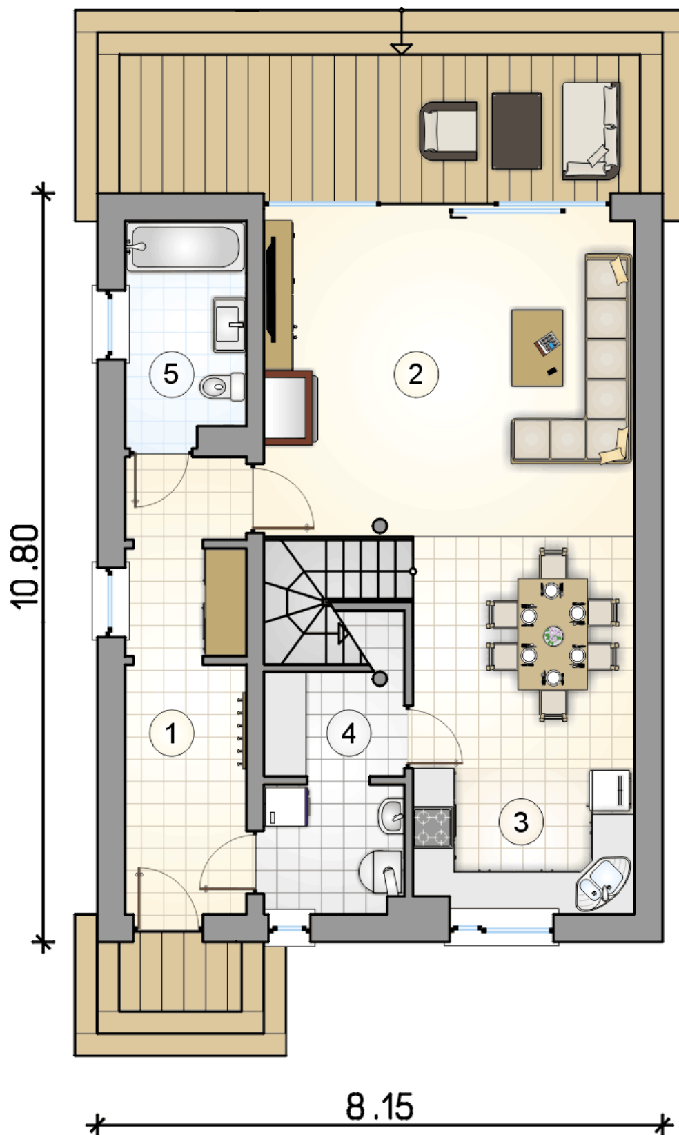
RZUT PARTERU
