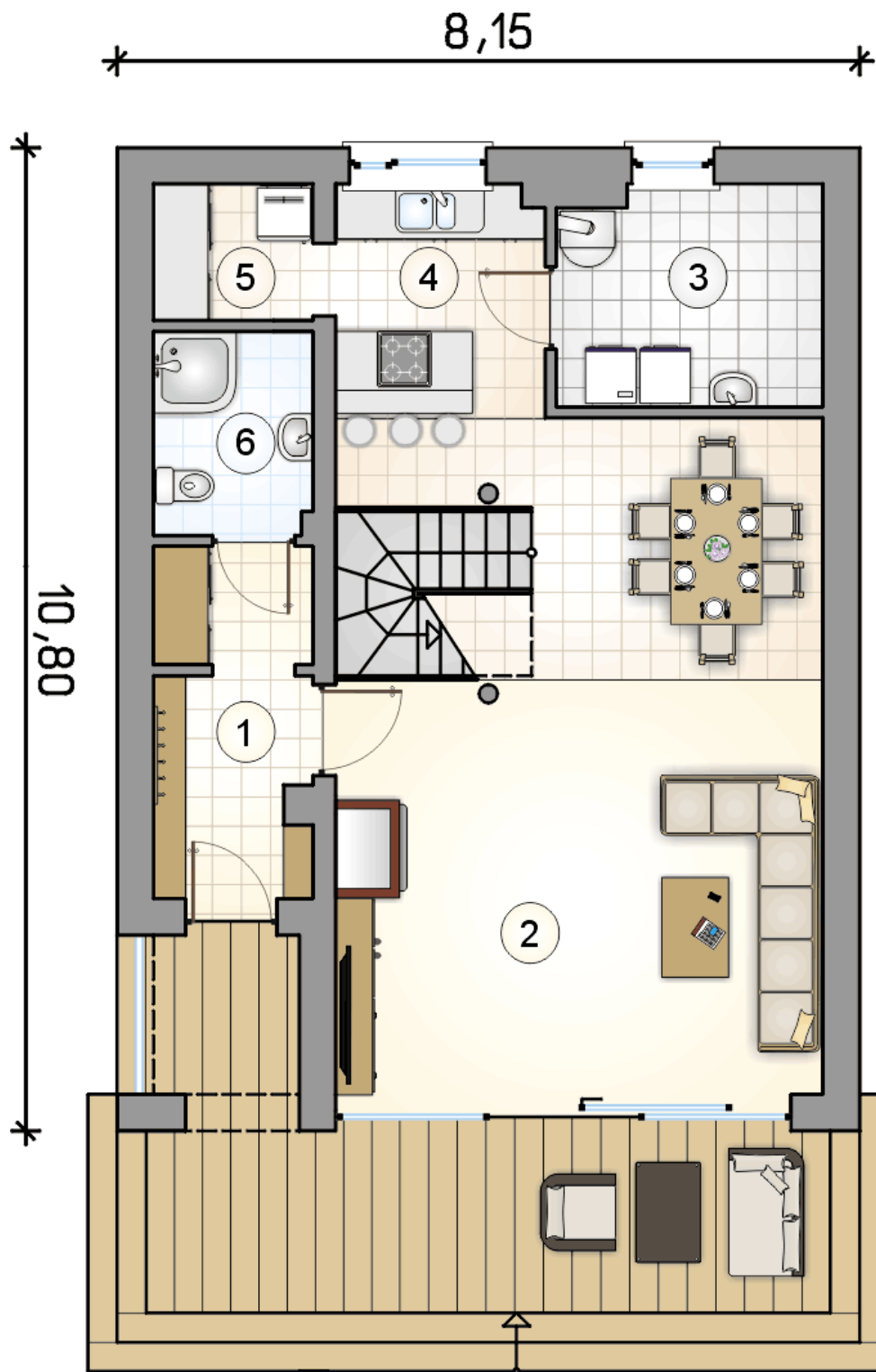
RZUT PARTERU
