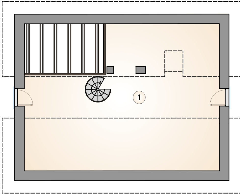
RZUT PODDASZA
