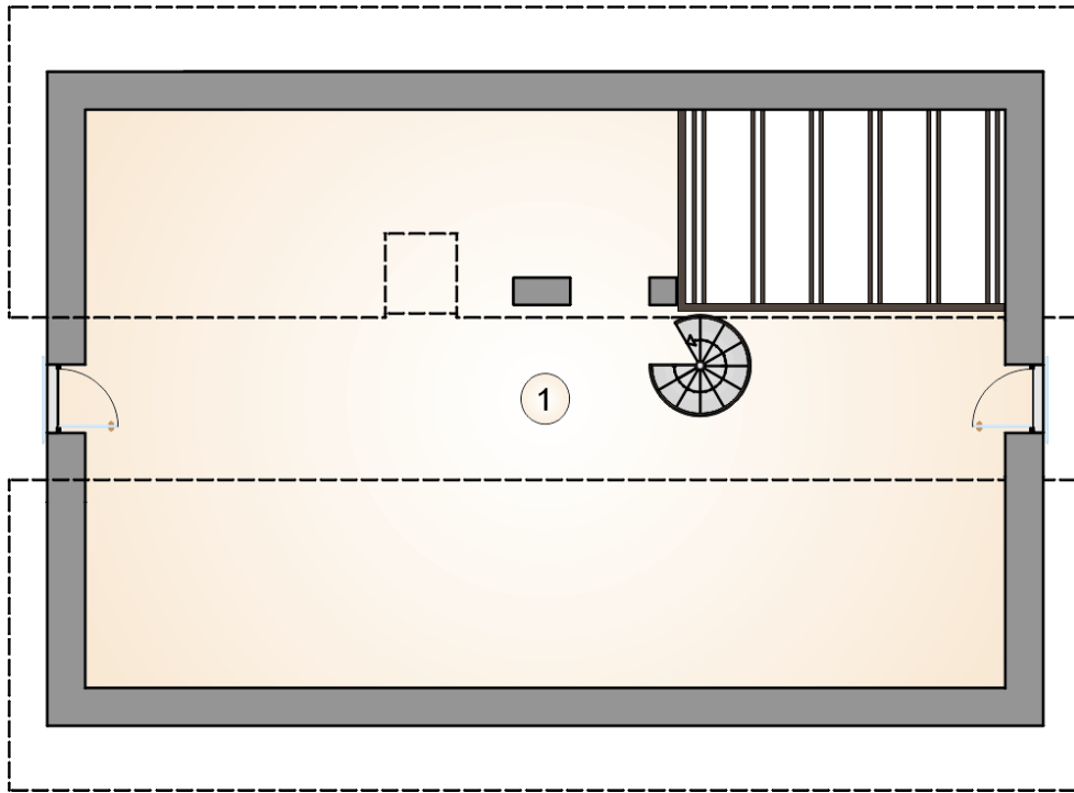
RZUT PODDASZA
