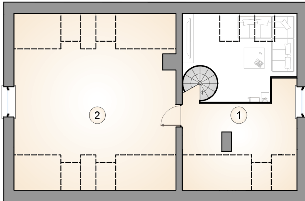
RZUT PODDASZA
