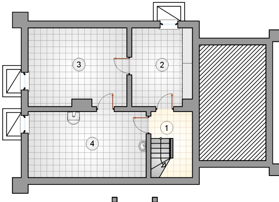
RZUT PIWNICY
