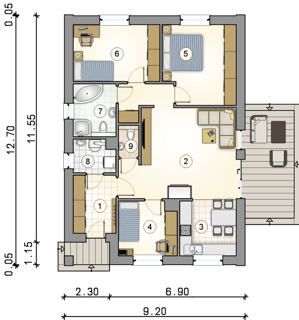
RZUT PARTERU
